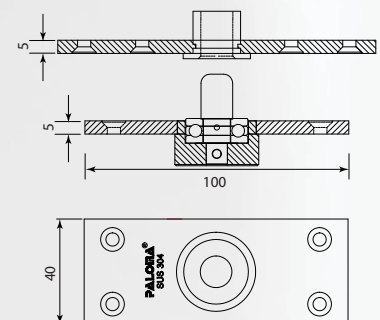
Bottom Pivot
