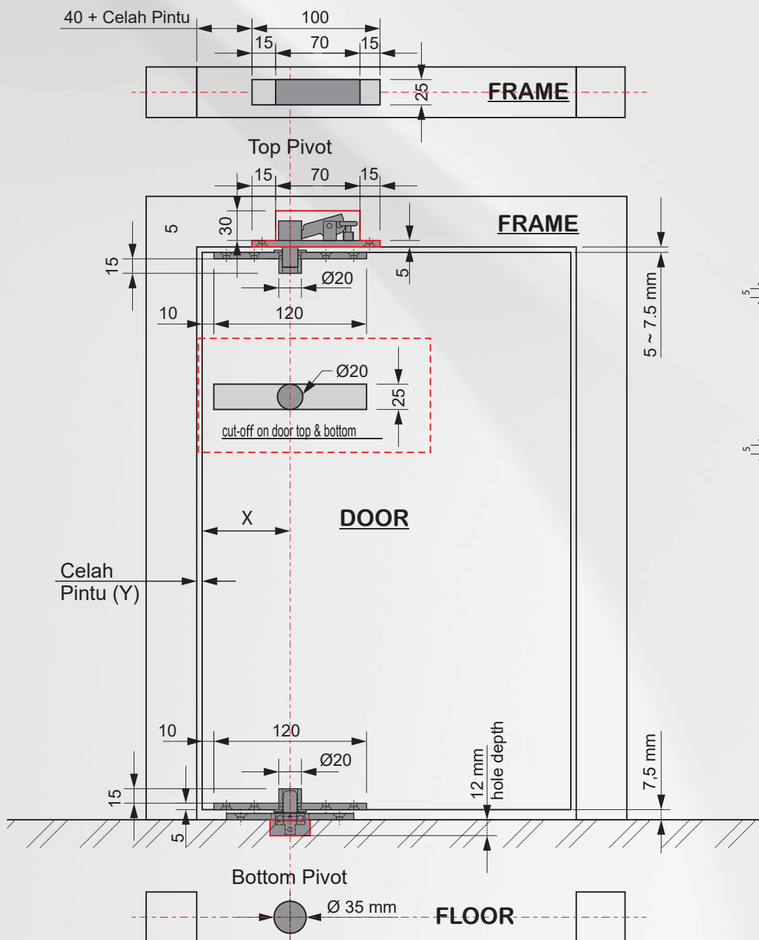
Bottom Pivot
